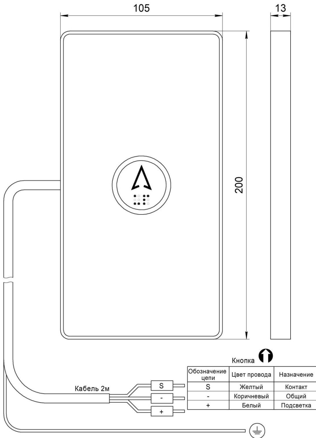
Рис.1 Внешний вид и габаритные размеры Вызывного поста МАЛАХИТ НШЕК.468381.061-01
